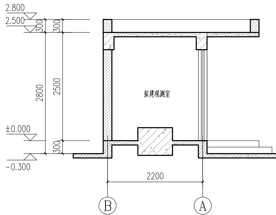
1-1剖面图 1:50
