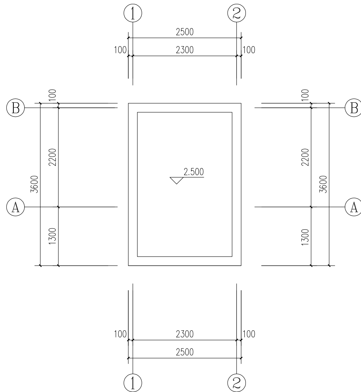
屋面平面图 1:50
