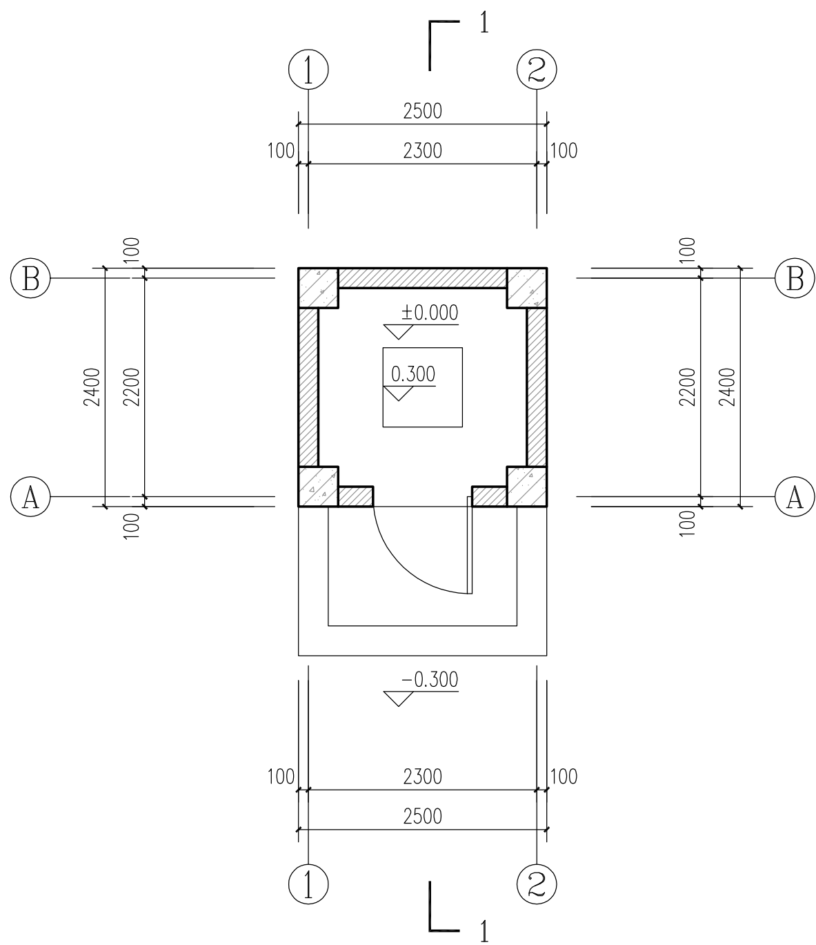
一层平面图 1:50
