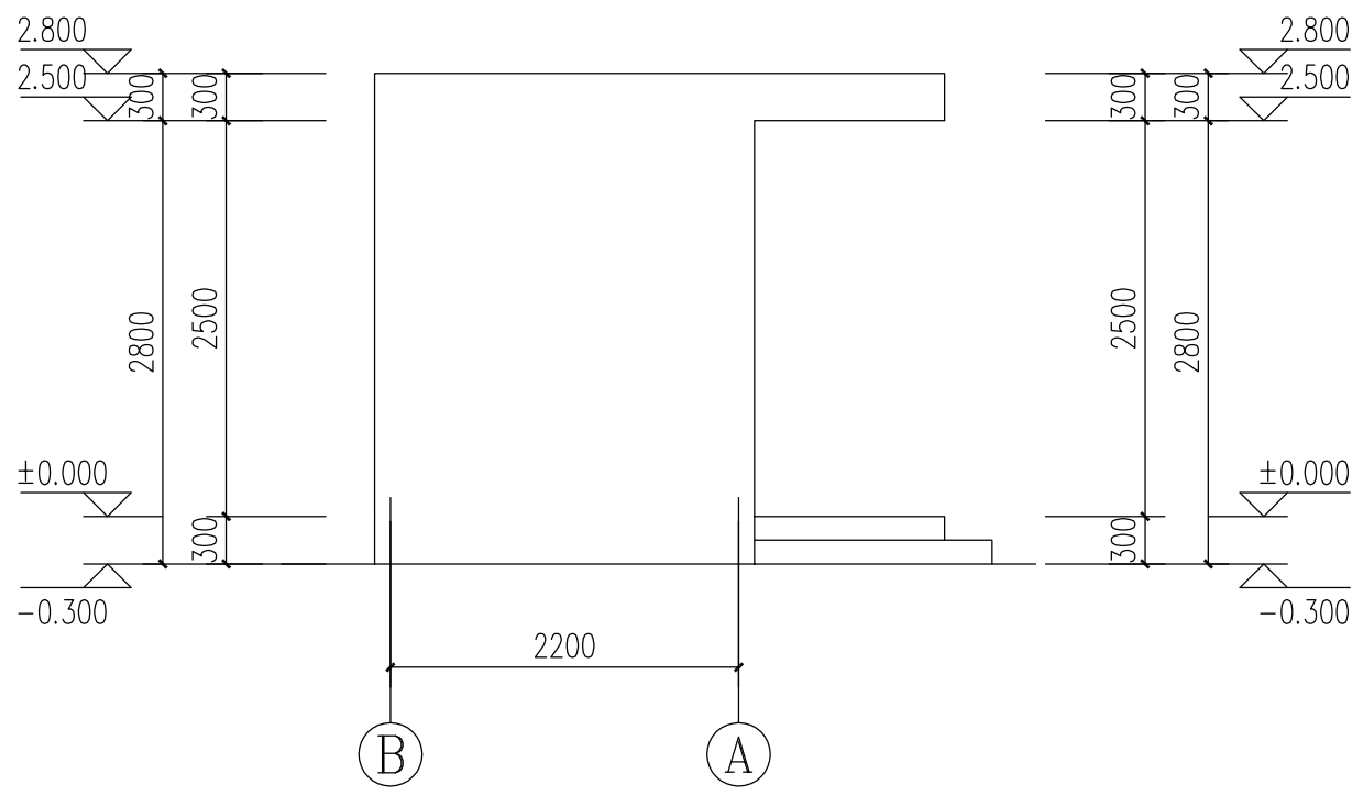
①-②立面图 1:50
