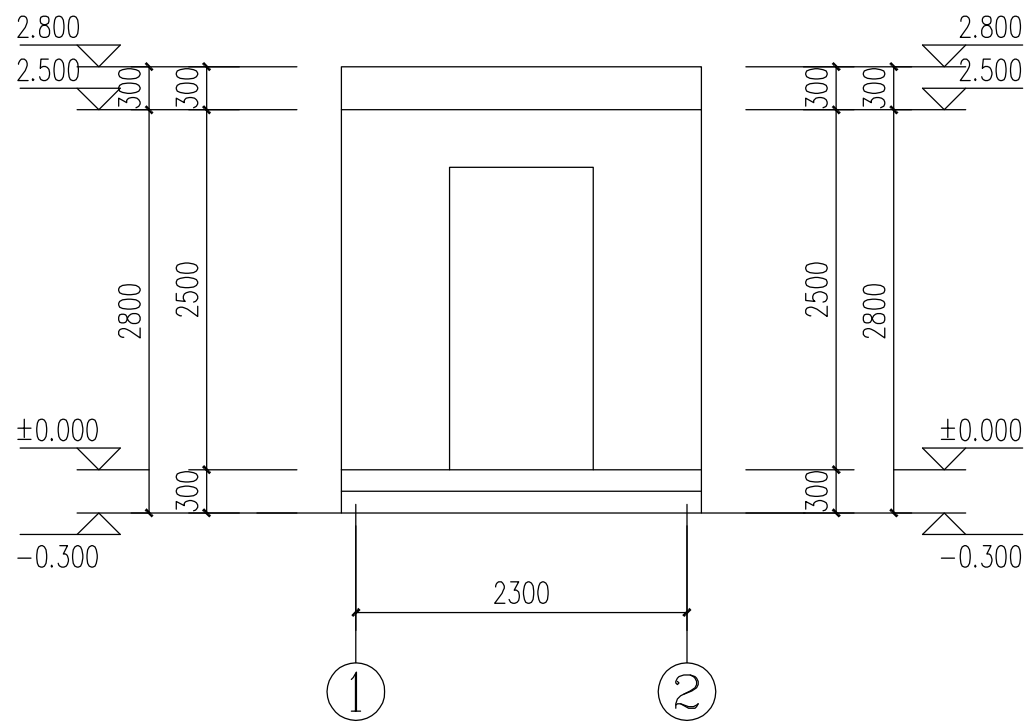
①-②立面图 1:50
